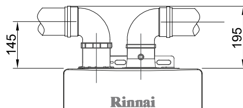
Tubos separados Ø 80-80
