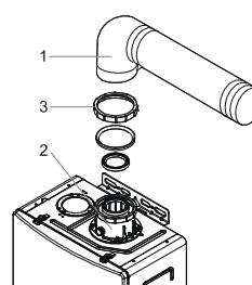
Tubos separados Ø 80-80
