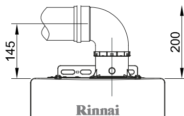
Tubos concéntricos Ø 60/100
